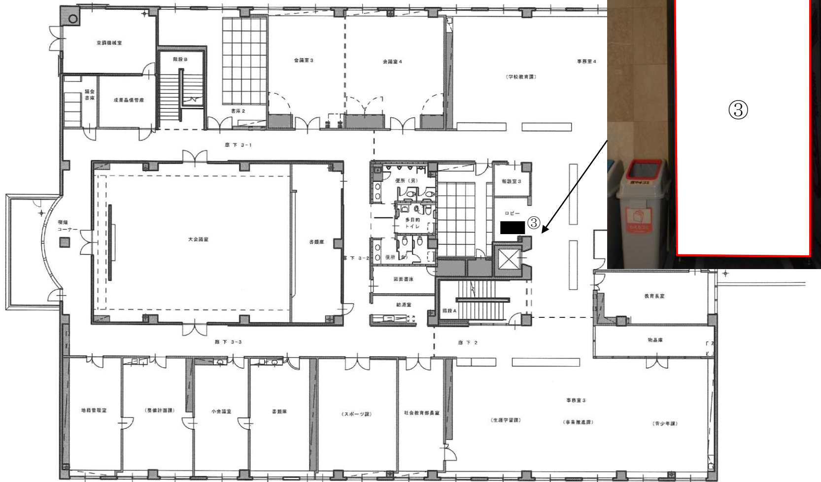
図面 1 6 端野総合支所 (2階) (北見市端野町二区471番地1)
